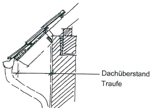
Skizze – Traufe für ein Pfettendach
