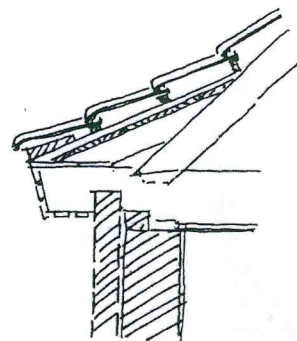
Skizze – Traufe für ein Kehlbalkendach
